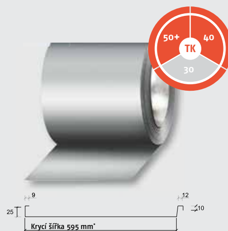
RUUKKI FALCOVACÍ SVITKY PLX (0,6mm ocel) a Emka (0,8mm hliník)
