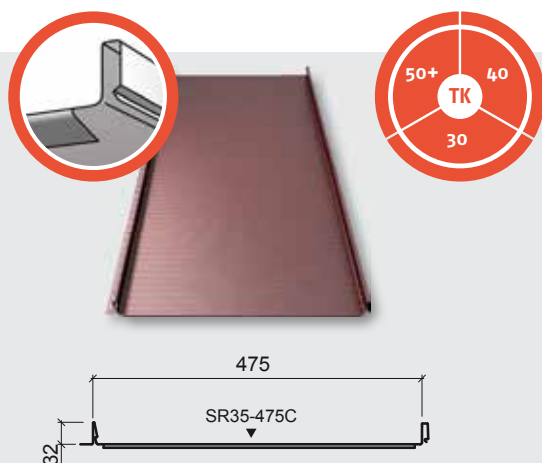
Ruukki CLASSIC C
