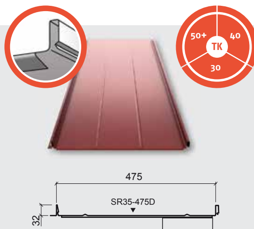
Ruukki CLASSIC D
